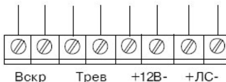
Блок обработки сигнала (БОС)
