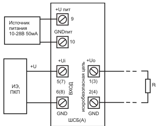
Рис.3 – Клеммные соединения барьера ШСБ(А).
