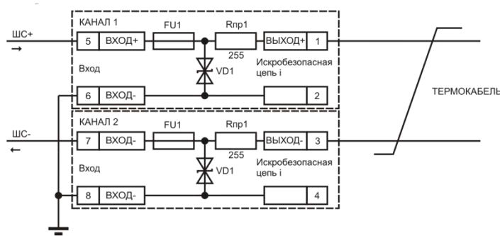
Рис.1 – Эквивалентная схема барьера ШСБ-ТК
