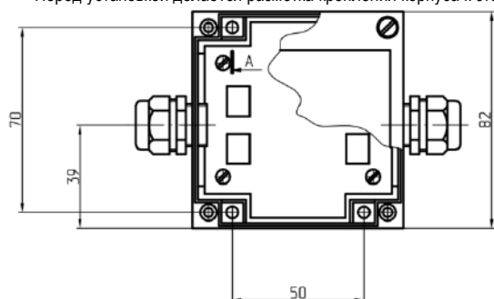
Рис.2 – Установочные размеры настенного исполнения ШСБ.
