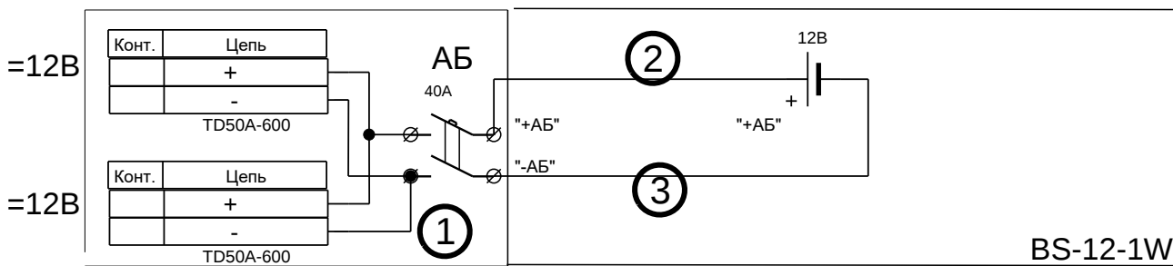
Рисунок 1.2 – Батарейный стеллаж Штиль BS-12-1W.
