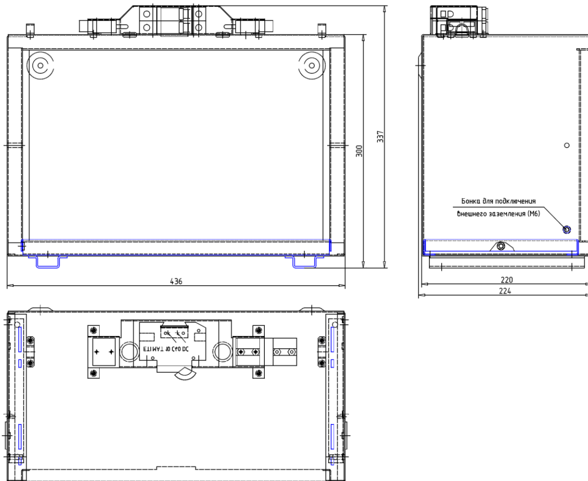
Рисунок 1.1 – Батарейный стеллаж Штиль BS-12-1W.
