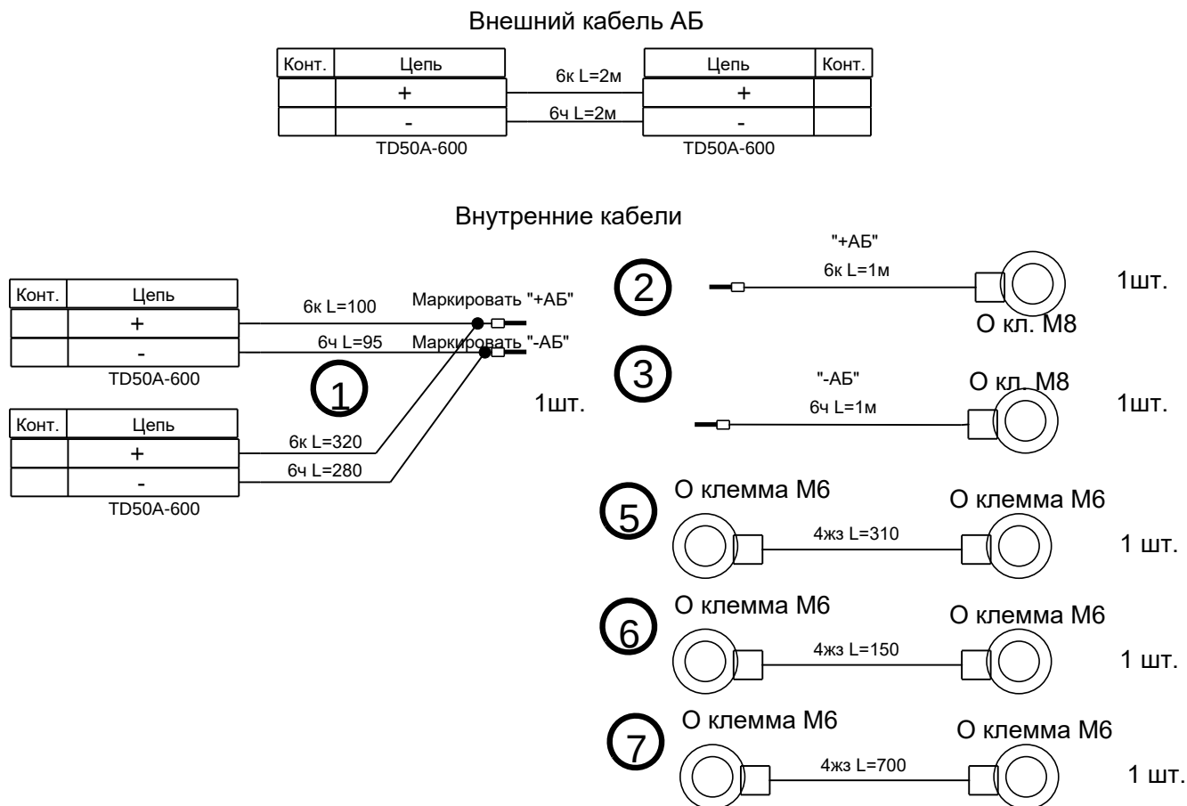
Рисунок 1.3 – Комплект кабелей к батарейному стеллажу Штиль BS-12-2W
