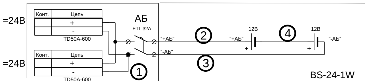
Рисунок 1.2 – Батарейный стеллаж Штиль BS-24-1W.
