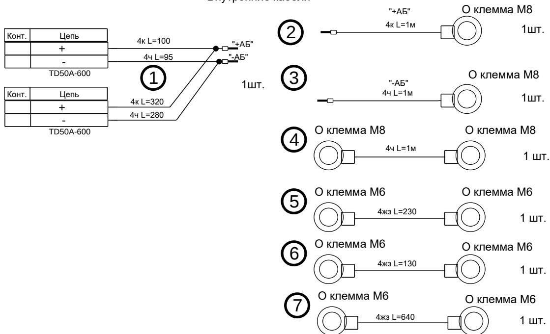
Рисунок 1.3 – Комплект кабелей к батарейному стеллажу Штиль BS-24-1W
