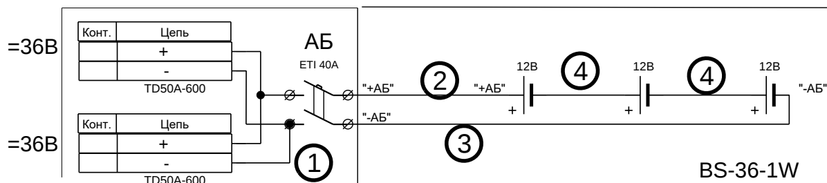
Рисунок 1.2 – Батарейный стеллаж Штиль BS-36-1W.
