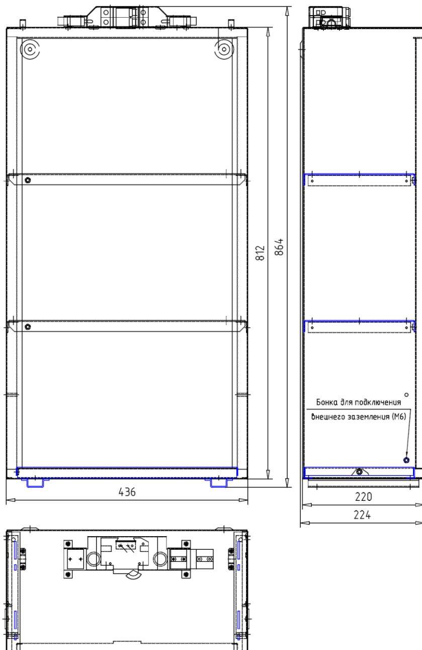
Рисунок 1.1 – Батареный стеллаж ШТИЛЬ BS-36-1W. Внешний вид и габариты изделия
