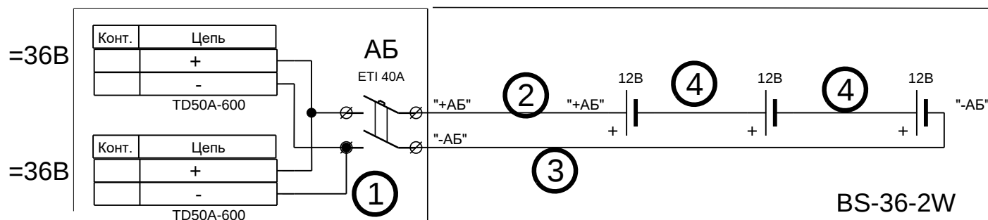
Рисунок 1.2 – Батарейный стеллаж Штиль BS-36-2W.
