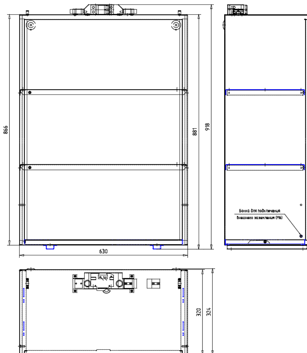
Рисунок 1.1 – Батарейный стеллаж Штиль BS-36-2W. Внешний вид и габариты изделия
