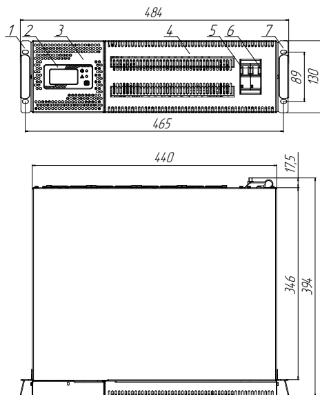
Рисунок 5а. Габаритные размеры и компоненты стабилизатора Штиль IS7000RT (горизонтальная установка)
