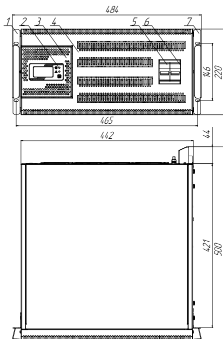
Рисунок 8а. Габаритные размеры и компоненты стабилизатора Штиль IS15000RT (горизонтальная установка)
