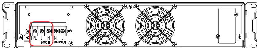
Рисунок 23. Стабилизатор Штиль IS5000RT. Выводы «Вход PE-L-N»
