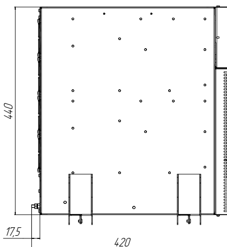
Рисунок 6б. Габаритные размеры и компоненты стабилизаторов Штиль IS8000RT и IS10000RT (вертикальная напольная установка)
