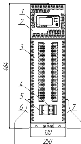
Рисунок 6б. Габаритные размеры и компоненты стабилизаторов Штиль IS8000RT и IS10000RT (вертикальная напольная установка)
