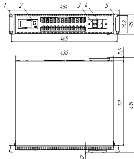
Рисунок 4а. Габаритные размеры и компоненты стабилизатора Штиль IS5000RT (горизонтальная установка)
