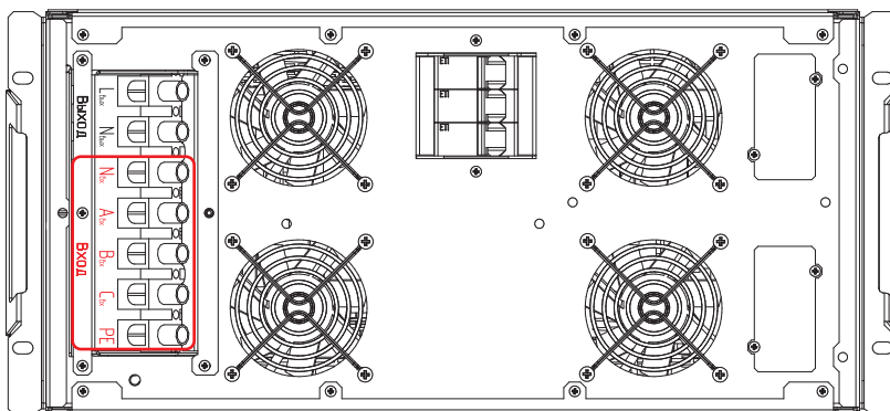
Рисунок 17б. Стабилизаторы IS3115RT и IS3120RT. Выводы «Вход Nвх-Авх-Ввх-Свх-РЕ»
