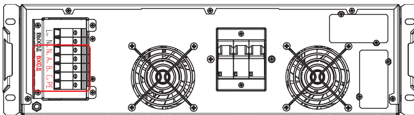
Рисунок 17а. Стабилизаторы IS3106RT, IS3108RT и IS3110RT. Выводы «Вход Nвх-Авх-Ввх-Свх-РЕ»
