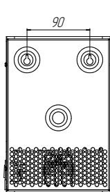
Рисунок 12а. Задняя панель стабилизатора Штиль IS350
