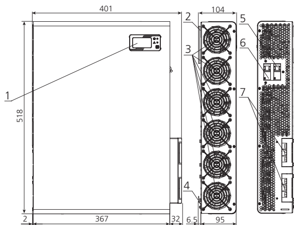
Рисунок 26. Габаритные размеры, компоненты передней и боковых панелей стабилизатора Штиль IS10000
