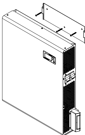
Рисунок 26. Крепление стабилизатора IS15000 на ровной вертикальной поверхности
