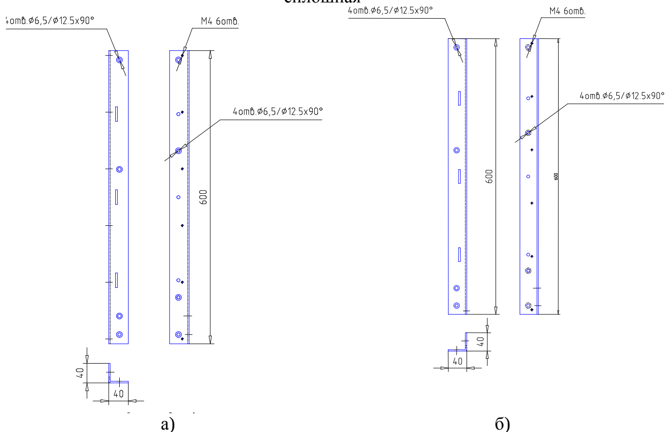
Рисунок 3.2 (б) – Батарейный стеллаж Штиль MBS-01. Стенка боковая СПЛОШНАЯ
