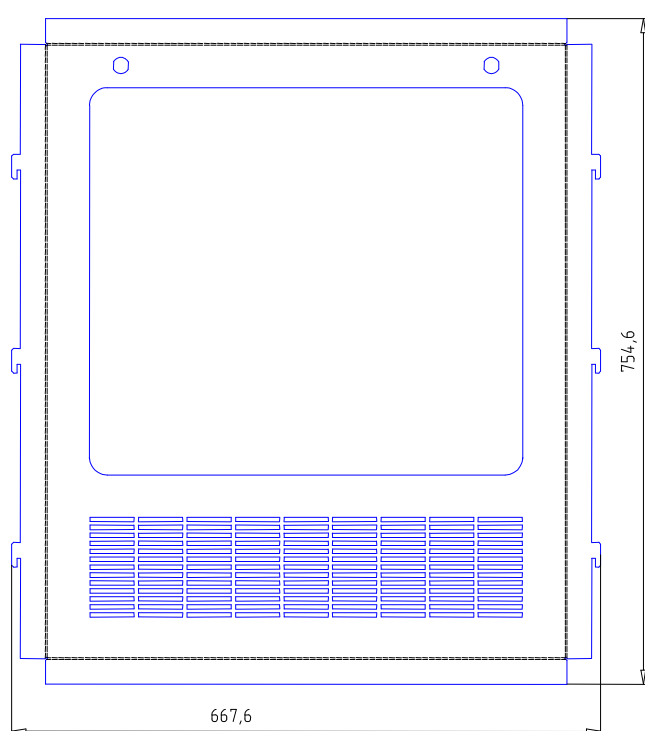
а) б) Рисунок 3.3 – Батарейный стеллаж Штиль MBS-02. а) - стенка передняя, б) - стенка задняя
