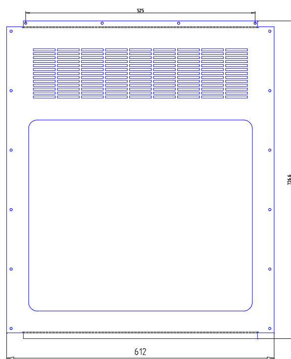
а) б) Рисунок 3.3 – Батарейный стеллаж Штиль MBS-02. а) - стенка передняя, б) - стенка задняя
