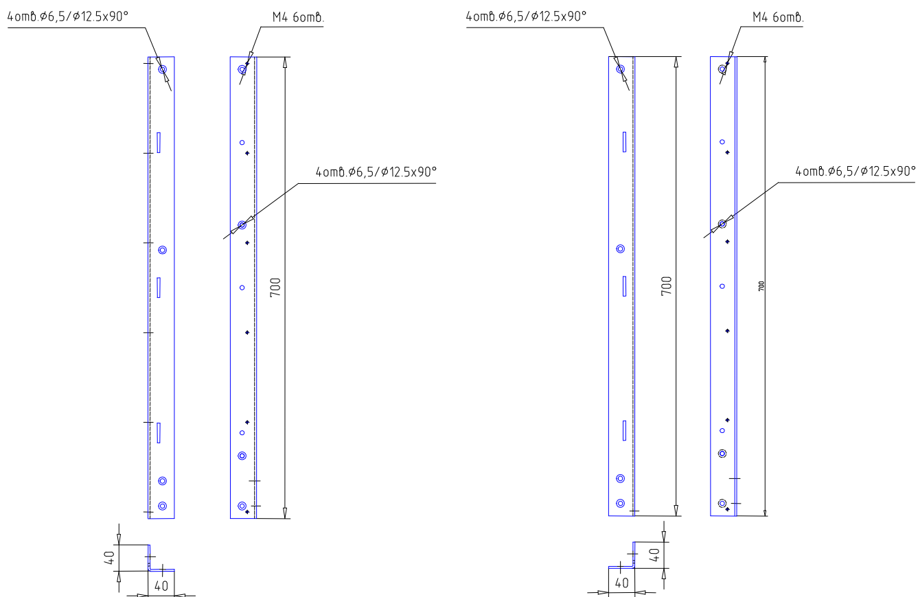
Рисунок 3.4 – Батарейный стеллаж Штиль МBS-02. а) - стойка передняя левая, б) - стойка передняя правая
