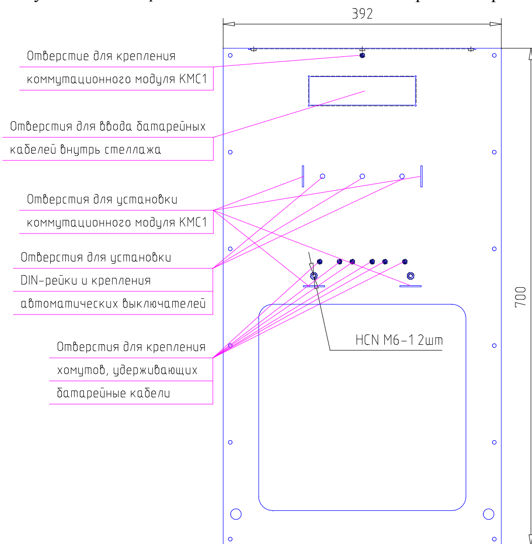
Рисунок 3.2 (а) – Батарейный стеллаж Штиль MBS-02. Стенка боковая с отверстиями
