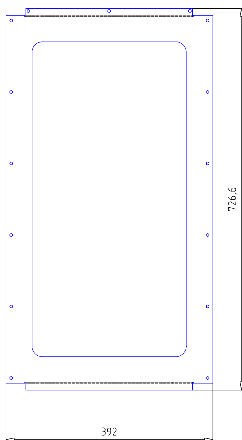
Рисунок 3.2 (б) – Батарейный стеллаж Штиль MBS-02. Стенка боковая СПЛОШНАЯ
