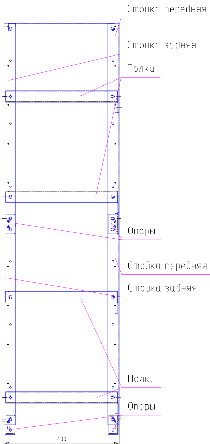
Рисунок 4.6 – Вид двух собранных и соединенных стеллажей MBS-03.
