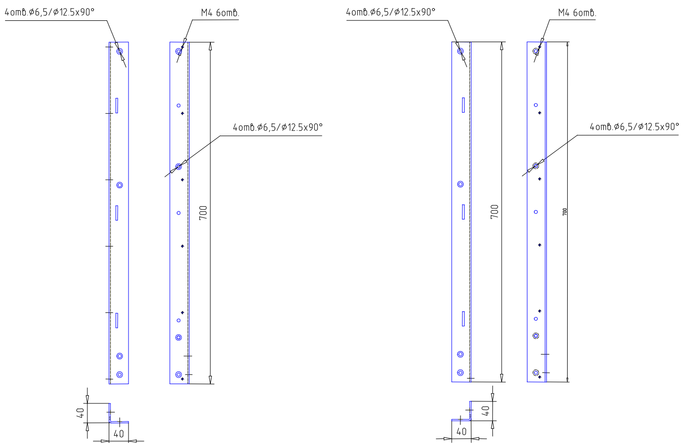
а) б) Рисунок 3.4 – Батарейный стеллаж Штиль MBS-03. а) - стойка передняя левая, б) - стойка передняя правая
