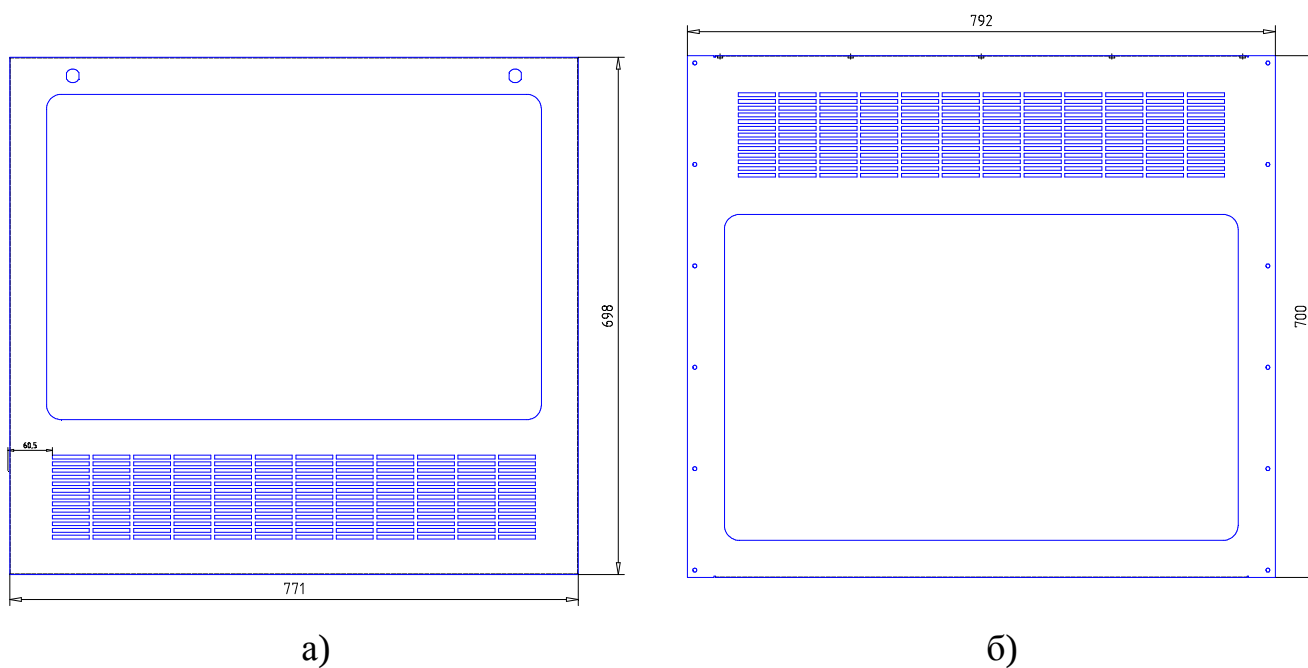
Рисунок 3.3 – Батарейный стеллаж Штиль MBS-03. а) - стенка передняя, б) - стенка задняя
