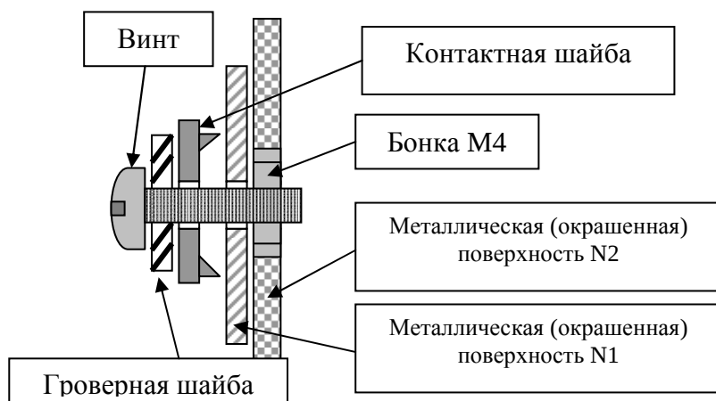
Рисунок – 5.3а Соединение: винт+гайка Рисунок 5.3в - Соединение: шпилька+гайка
