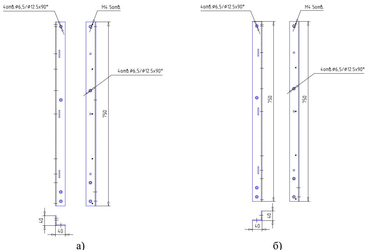
Рисунок 3.3 – Батарейный стеллаж Штиль MBS-04. а) - стойка передняя левая, б) - стойка передняя правая
