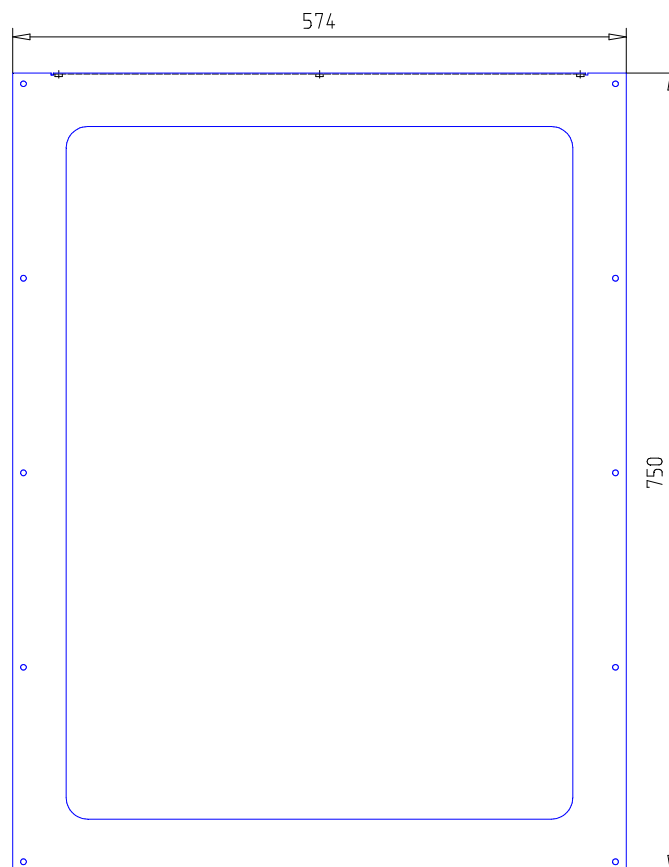
Рисунок 3.2 (б) – Батарейный стеллаж Штиль MBS-04. Стенка боковая СПЛОШНАЯ
