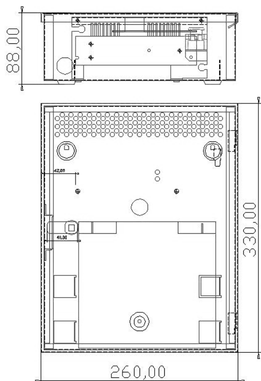
Рисунок 1.1 – Внешний вид ИБП Штиль PS2405D
