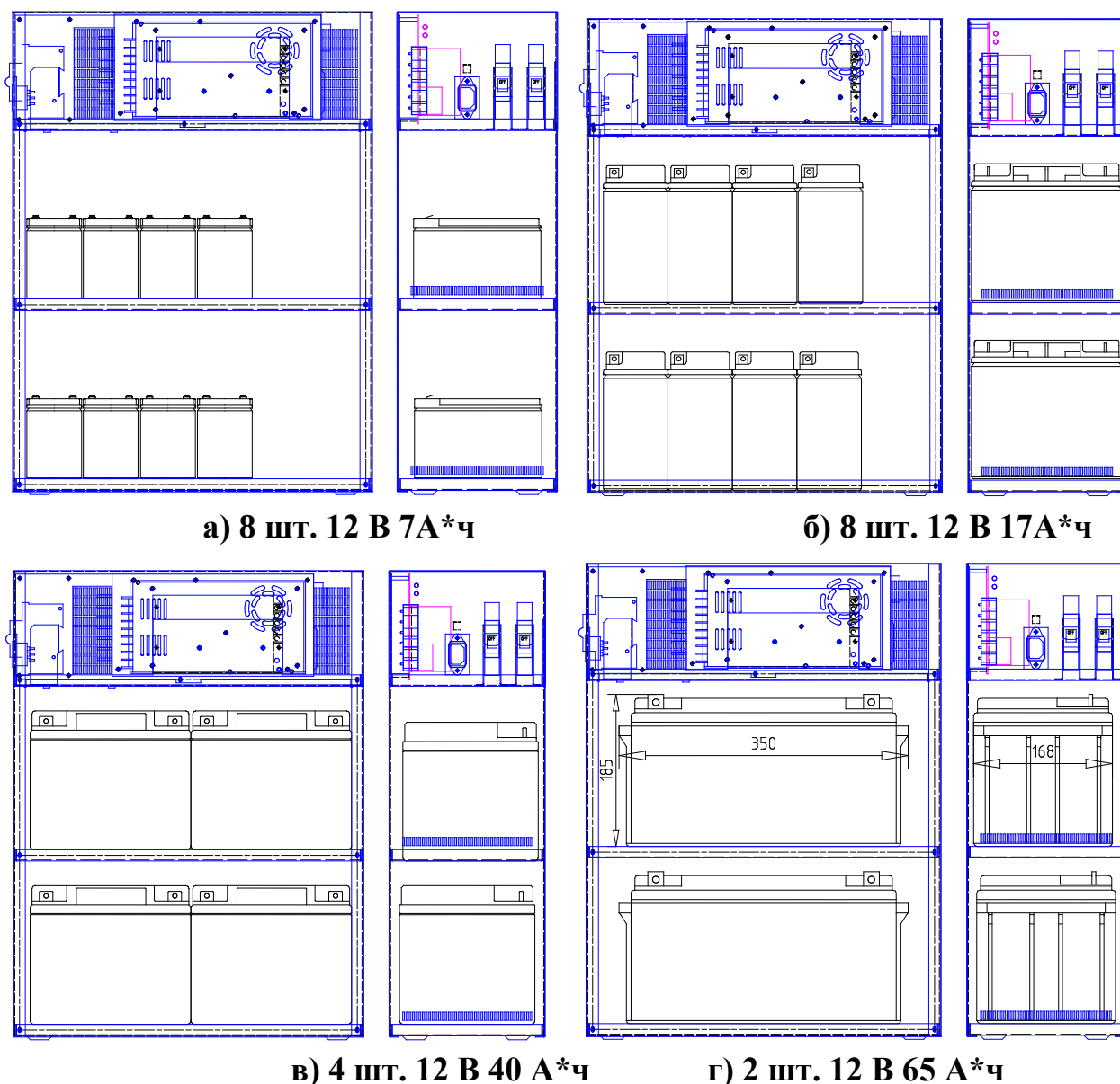
Рисунок 2.2 – Пример расположения АБ в ИБП Штиль
