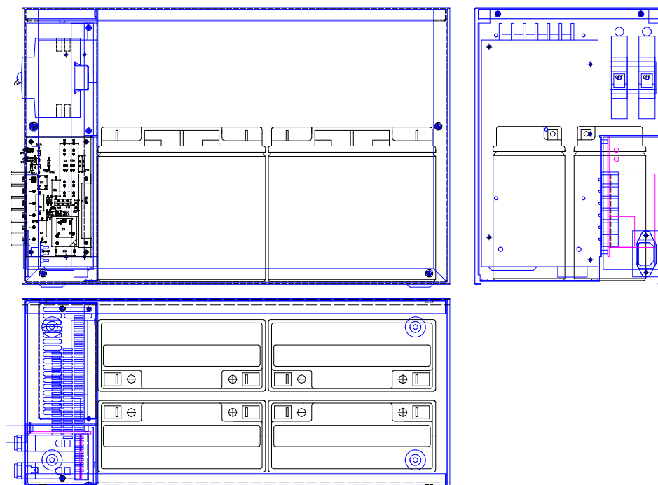
Рисунок 2.4 – Пример расположения АБ (4 шт. 12 В 17А*ч ) в ИБП Штиль PS4805G и PS4810G
