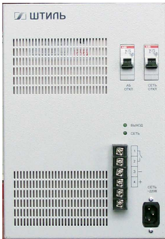
Рисунок 1.2 – Внешний вид ИБП Штиль PS4805G, PS4810G а) габаритные размеры; б) внешний вид, в) внешний вид изделий в модификации с «холодным пуском»
