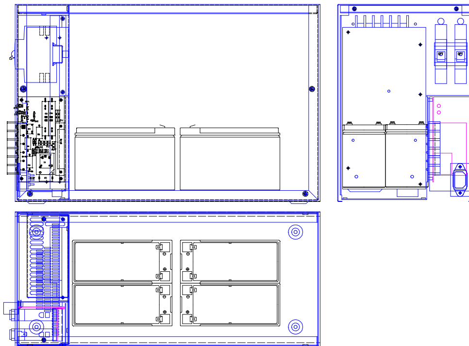
Рисунок 2.3 – Пример расположения АБ (4 шт. 12 В 7А*ч ) в ИБП Штиль PS4805G и PS4810G
