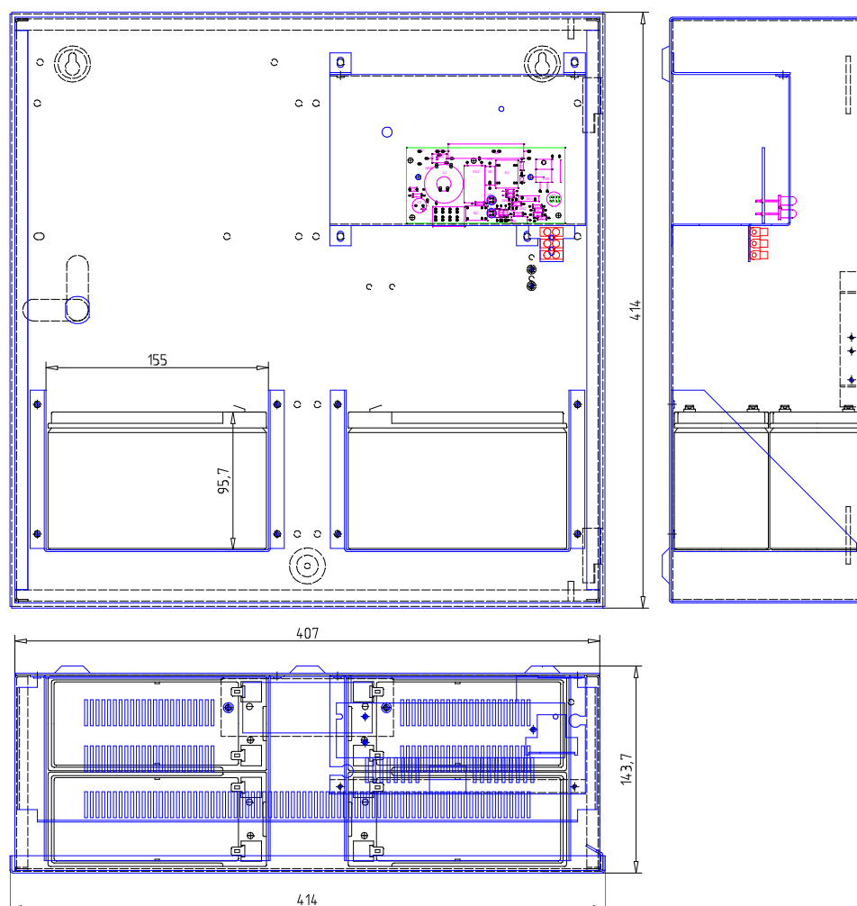
Рисунок 2.2 – Пример расположения АБ в ИБП Штиль PS4802Е (4 шт. 12 В 7А*ч)
