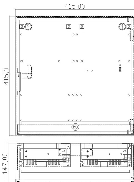
а) б) Рисунок 1.1 – Внешний вид ИБП Штиль PS4802E а) габаритные размеры; б) внешний вид
