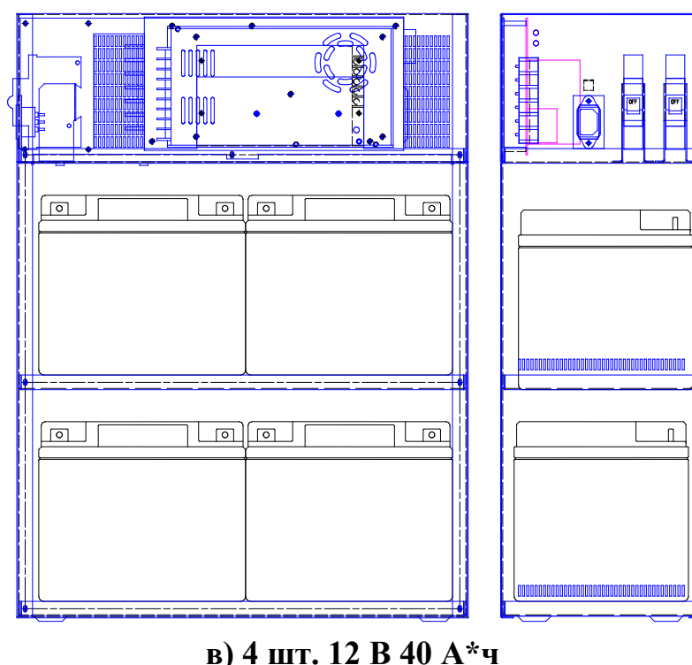
Рисунок 2.2 – Пример расположения АБ в ИБП Штиль
