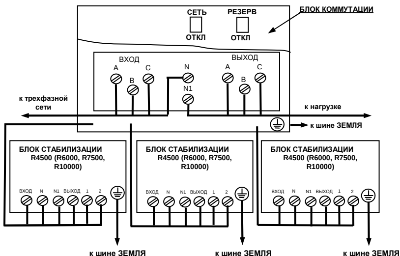
Рисунок 6.1 Схема подключения стабилизатора R13500-3 (R18000-3, R22500-3, R30000-3)
