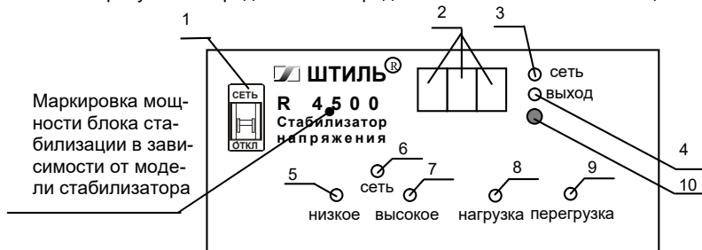
Рисунок 4.1 Передняя панель блока стабилизации
