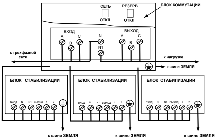
Рисунок 6.1 Схема подключения стабилизатора R13500-3 (R15000-3, R18000-3, R22500-3, R24000-3, R30000-3)
