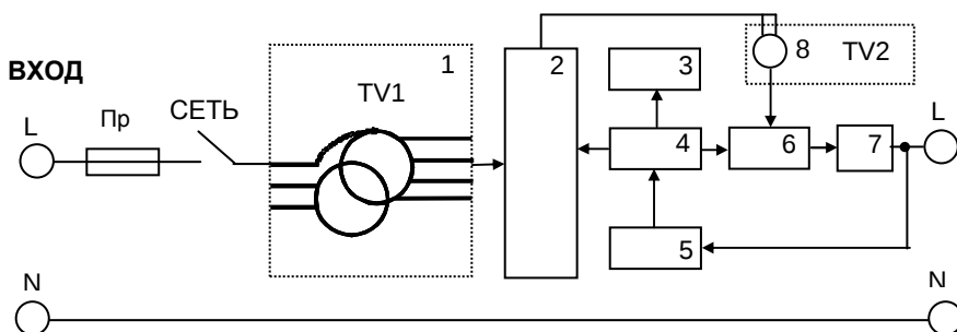
Рисунок 4.2 Структурно-функциональная схема стабилизатора
