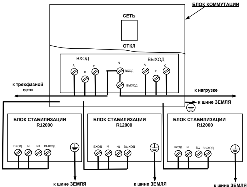
Рисунок 6.1 Схема подключения стабилизатора R36000-3
