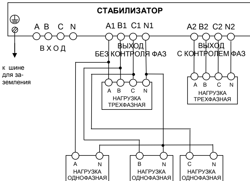
Рисунок 6.1 Схема подключения стабилизатора к сети и нагрузке
