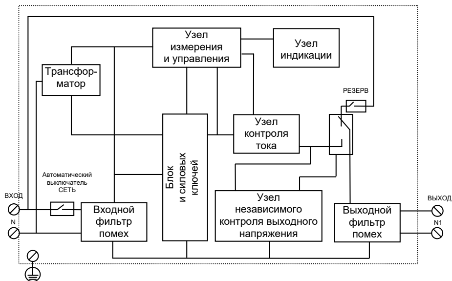
Рисунок 4.2 Функциональная схема стабилизатора
