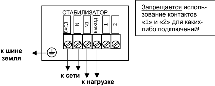
Рисунок 6.1 Схема подключения стабилизатора R4500C (R6000C, R7500C, R10000C, R12000C)
