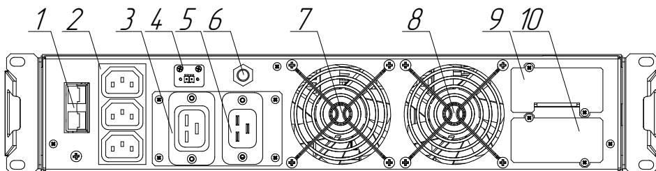
Рисунок 3б. Компоненты задней панели ИБП Штиль SR1102L и SR1103L
