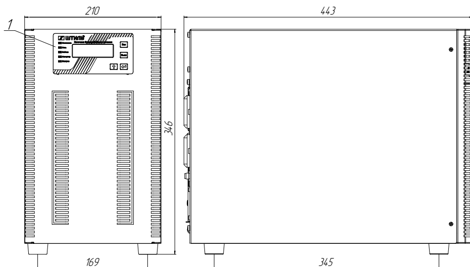
Рисунок 26. Габаритные размеры и компоненты передней панели ИБП Штиль ST1102SL, ST1102L, ST1103SL, ST1103L и ST1103TL
