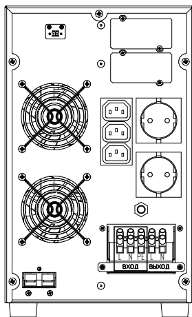
Рисунок 11. ИБП Штиль ST1103TL. Выводы «Вход L-N-PE»
