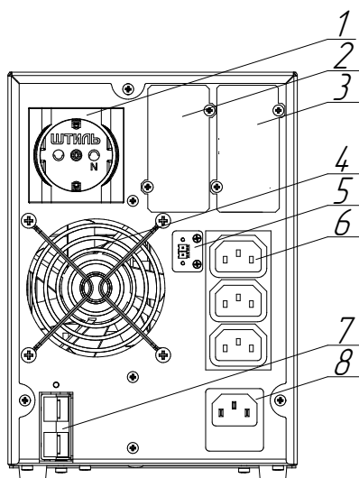
Рисунок 3а. Компоненты задней панели ИБП Штиль ST1101SL и ST1101L
