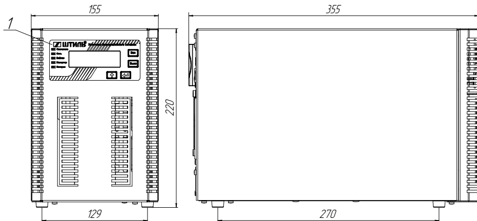
Рисунок 2а. Габаритные размеры и компоненты передней панели ИБП Штиль ST1101SL и ST1101L
