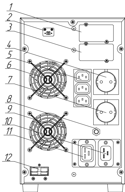
Рисунок 36. Компоненты задней панели ИБП Штиль ST1102SL, ST1102L, ST1103SL и ST1103L
