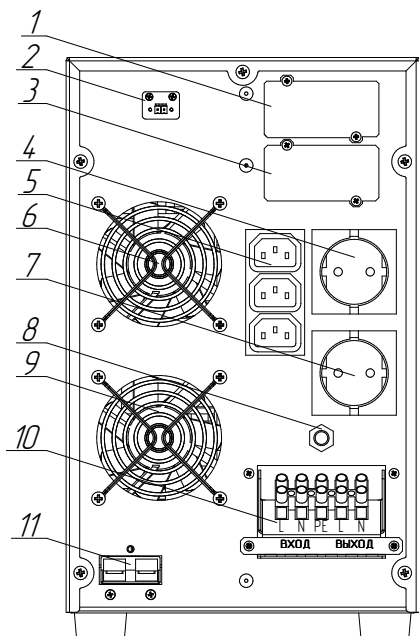
Рисунок 3в. Компоненты задней панели ИБП Штиль ST1103TL
