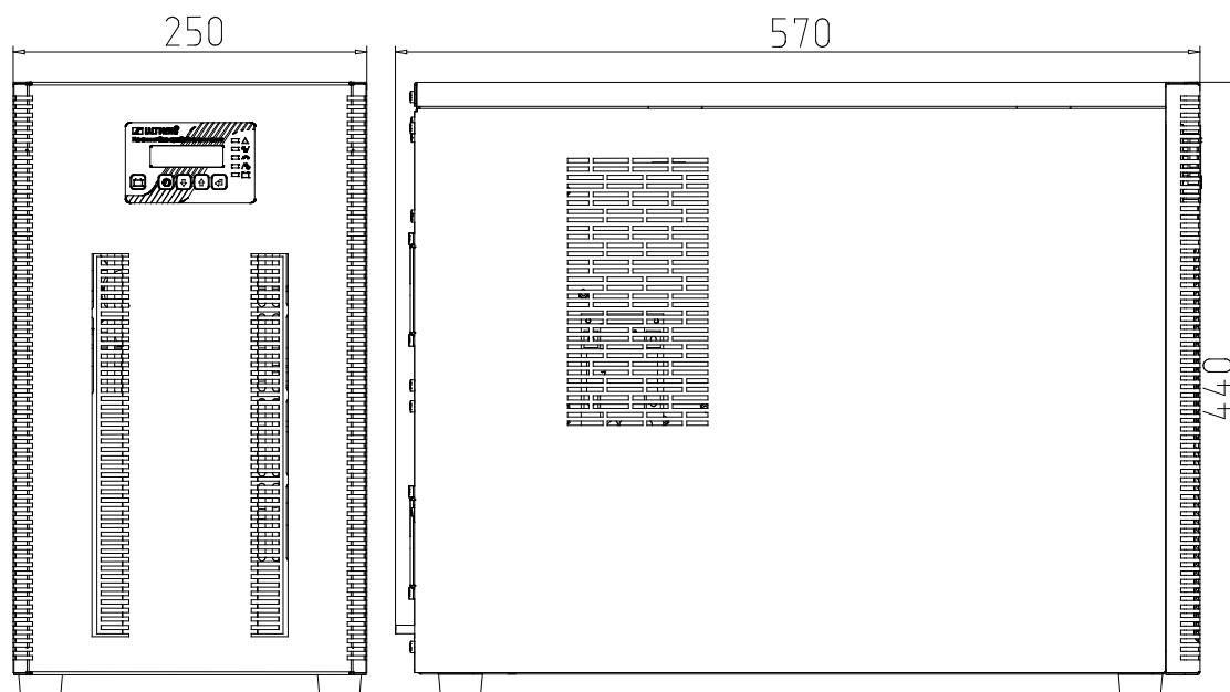
Рисунок 1.1 – ИБП Штиль ST1106L, ST1110L. Габаритные размеры и внешний вид
