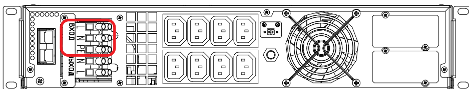
Рисунок 18б. ИБП Штиль STR1103TL. Выводы «Вход L-N-PE»
