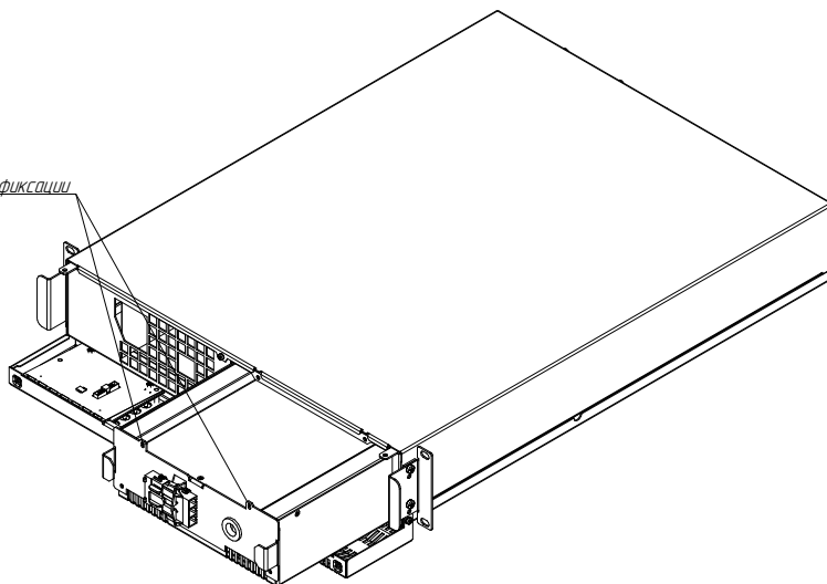
Рисунок Б3. Извлечение батарейного блока из ИБП Штиль STR1102SL и STR1103SL.
