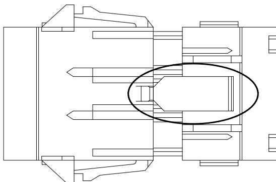
Рисунок Б1. Фиксатор батарейных разъёмов (ИБП Штиль STR1102SL и STR1103SL).
