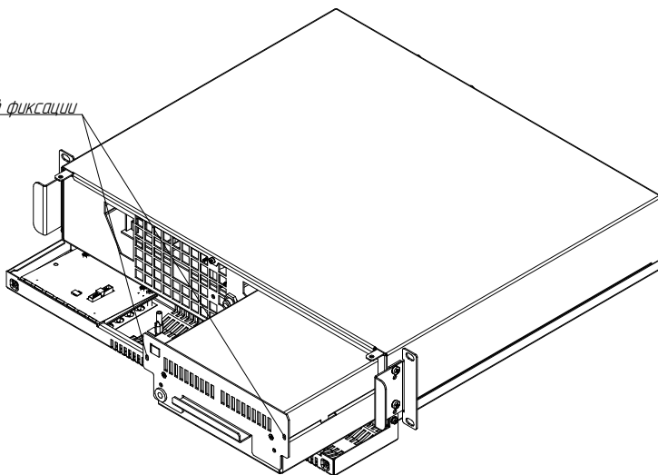
Рисунок Б2. Извлечение батарейного блока из ИБП Штиль STR1101SL.
