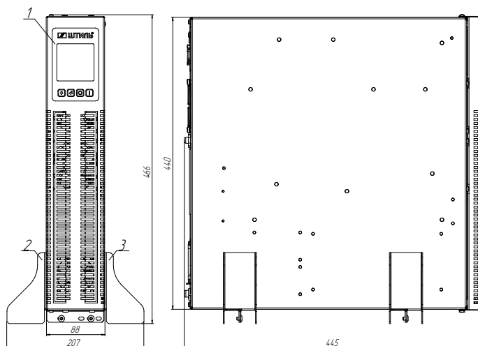
Рисунок 66. Габаритные размеры и компоненты ИБП Штиль STR1102L, STR1103L и STR1103TL (вертикальная напольная установка)
