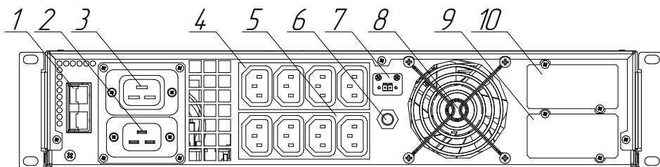
Рисунок 11. Компоненты задней панели ИБП Штиль STR1102L и STR1103L
