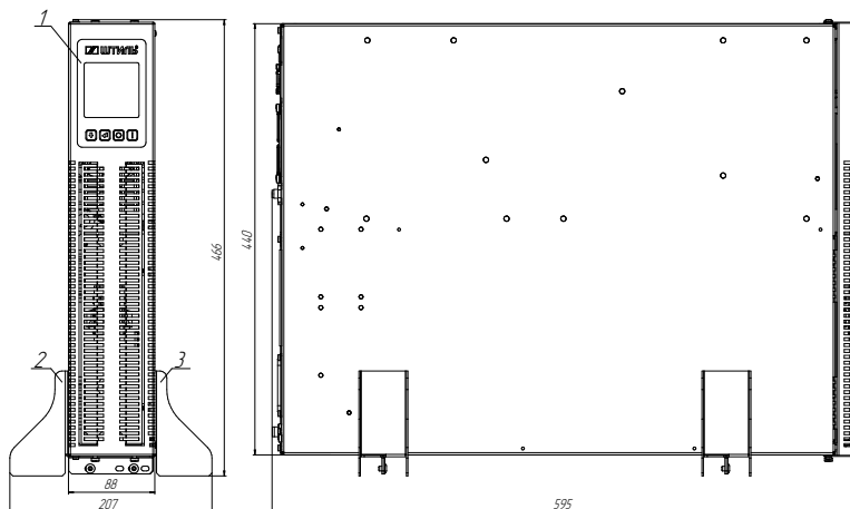
Рисунок 5б. Габаритные размеры и компоненты ИБП Штиль STR1102SL, STR1102LD, STR1103SL и STR1103TLD (вертикальная напольная установка)
