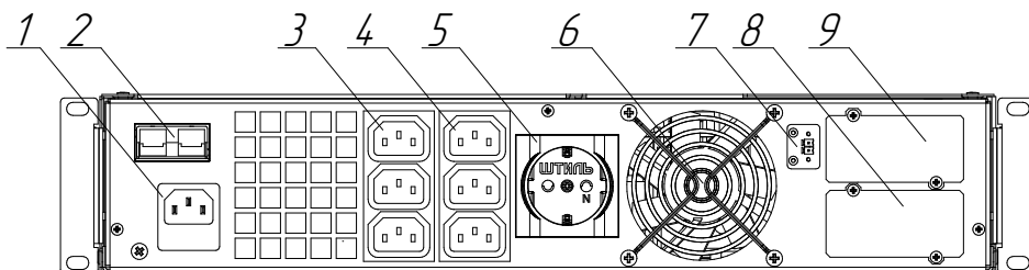
Рисунок 7. Компоненты задней панели ИБП Штиль STR1101L и STR1101SL
