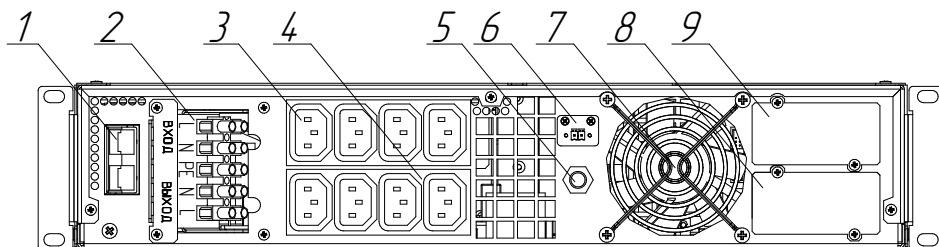
Рисунок 10. Компоненты задней панели ИБП Штиль STR1103TLD
