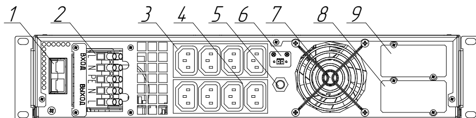
Рисунок 12. Компоненты задней панели ИБП Штиль STR1103TL
