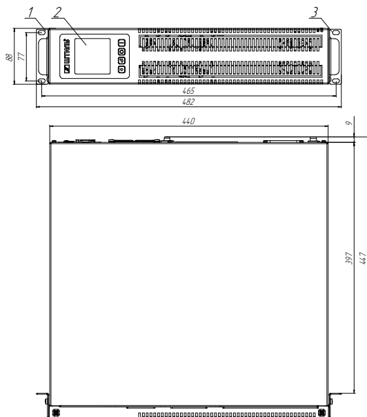
Рисунок 6а. Габаритные размеры и компоненты ИБП Штиль STR1102L, STR1103L и STR1103TL (горизонтальная установка в стойку)
