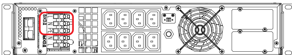
Рисунок 18б. ИБП Штиль STR1103TL. Выводы «Вход L-N-PE»
