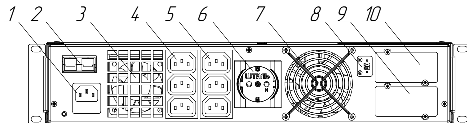
Рисунок 8. Компоненты задней панели ИБП Штиль STR1101LD
