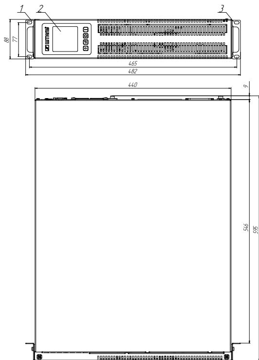
Рисунок 5а. Габаритные размеры и компоненты ИБП Штиль STR1102SL, STR1102LD, STR1103SL и STR1103TLD (горизонтальная установка в стойку)
