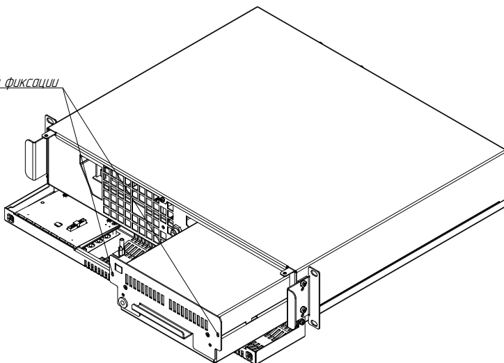
Рисунок Б1. Извлечение батарейного блока из ИБП Штиль STR1101SL.
