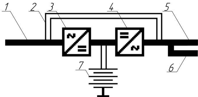
Рисунок 15. Компоненты мнемосхемы
