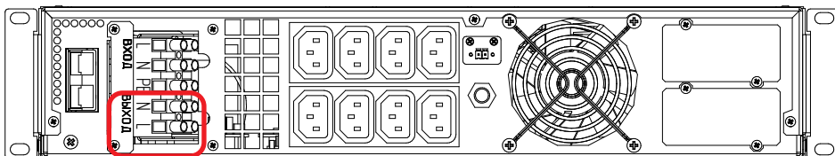
Рисунок 19б. ИБП Штиль STR1103TL. Выводы «Выход N-L»
