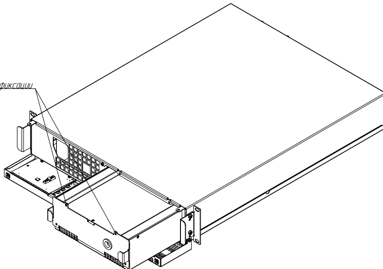
Рисунок Б2. Извлечение батарейного блока из ИБП Штиль STR1102SL и STR1103SL.
