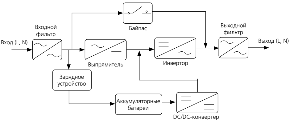
Рисунок 13. Структурная схема принципа работы ИБП
