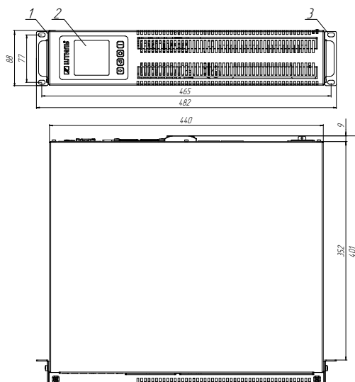
Рисунок 4а. Габаритные размеры и компоненты ИБП Штиль STR1101L, STR1101SL и STR1101LD (горизонтальная установка в стойку)
