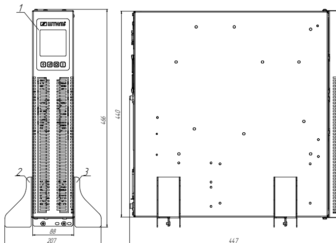
Рисунок 66. Габаритные размеры и компоненты ИБП Штиль STR1102L, STR1103L и STR1103TL (вертикальная напольная установка)
