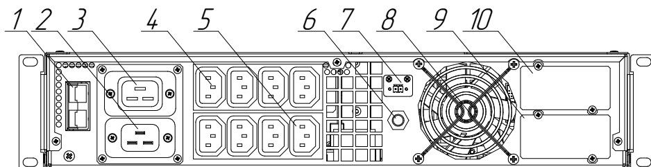
Рисунок 9. Компоненты задней панели ИБП Штиль STR1102SL, STR1102LD и STR1103SL
