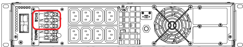
Рисунок 18а. ИБП Штиль STR1103TLD. Выводы «Вход L-N-PE»
