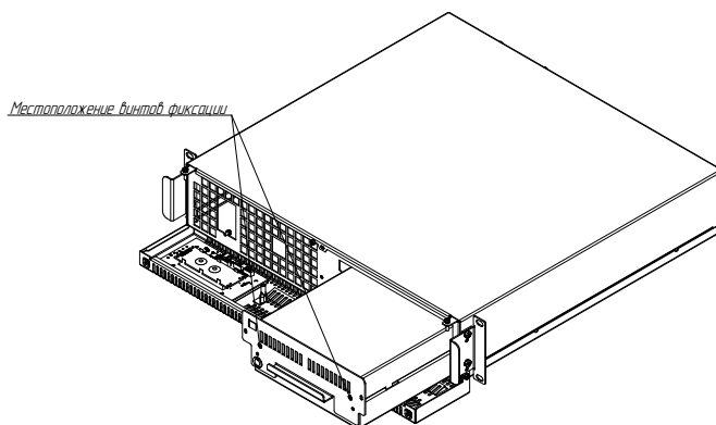
Рисунок Б2. Извлечение батарейного блока из ИБП Штиль STR500SL и STR500SL-18
