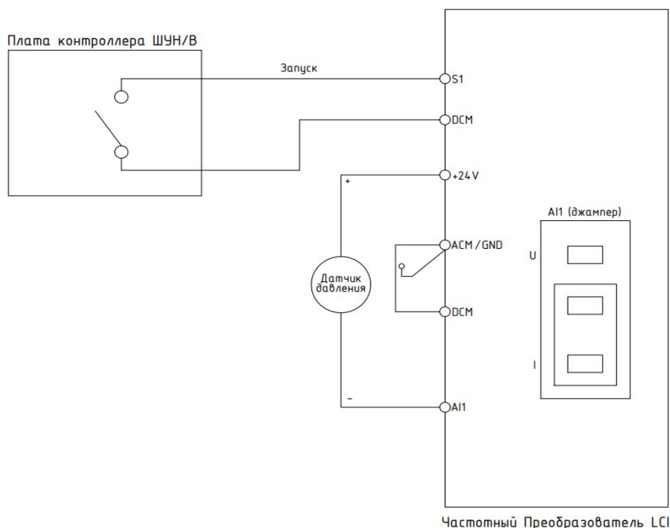
Схема подключения ШУН/В-ПЧ-R2 с аналоговым датчиком.
