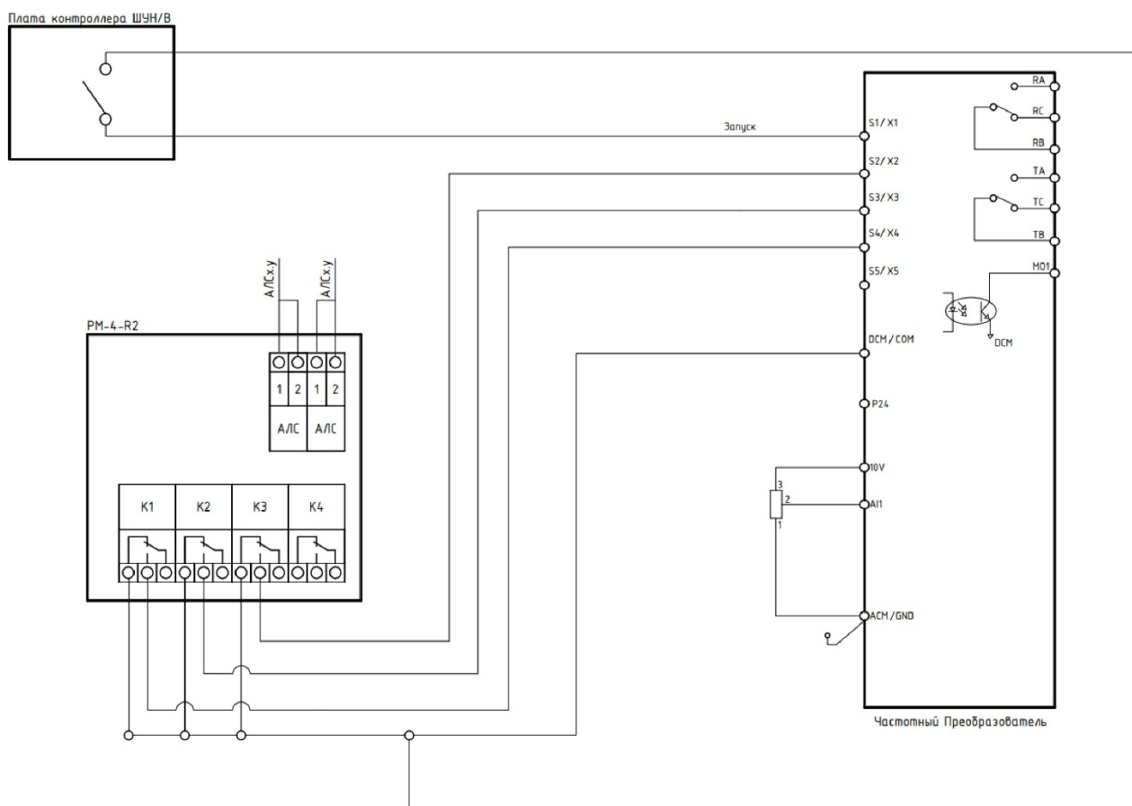
Схема подключения РМ-4-Р2 и частотного преобразователя Instart.
