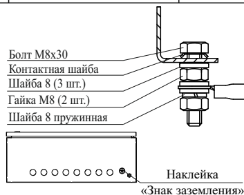
б) ШУ со степенью защиты оболочкой IP54
