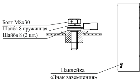
а) ШУ со степенью защиты оболочкой IP31
