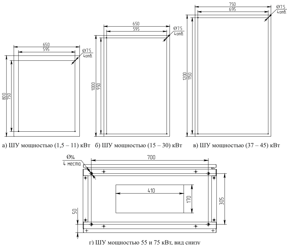
Рисунок 6 – Установочные размеры ШУ
