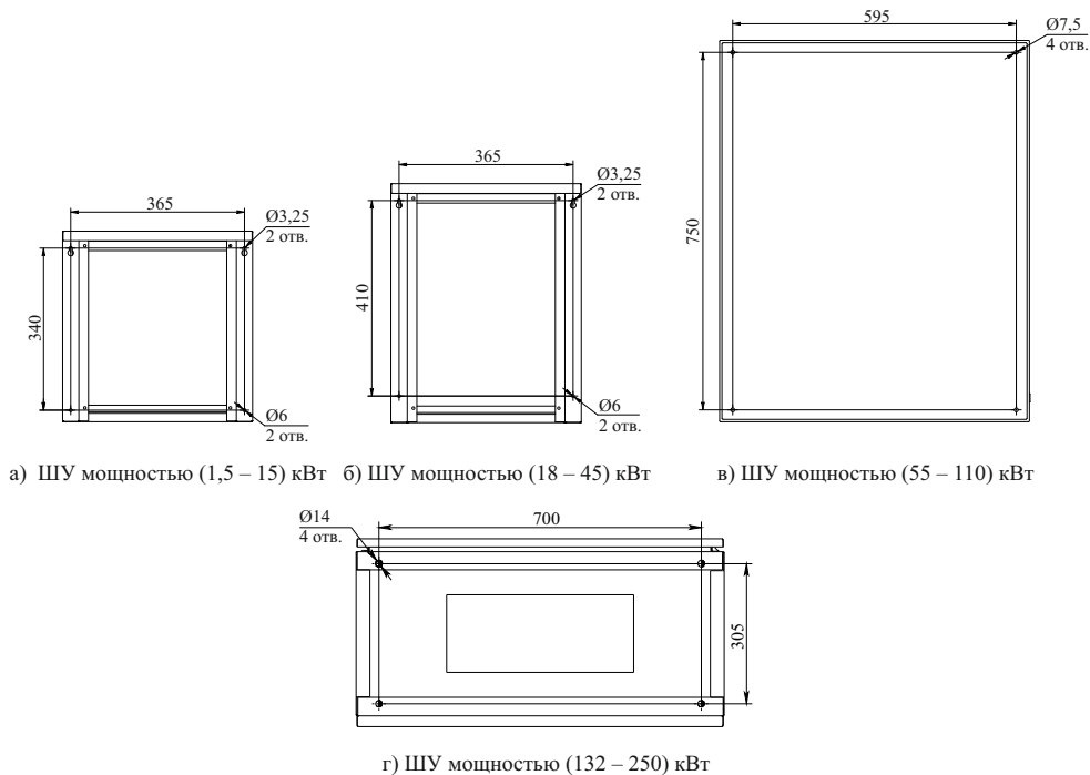
Рисунок 6 – Установочные размеры ШУ
