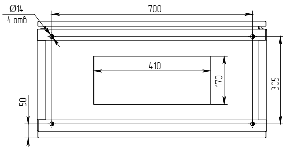
Рисунок 7 – Установочные размеры ШУ мощностью (90 – 250) кВт, вид снизу
