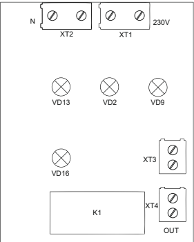
Рисунок 4 – Модуль контроля фаз
