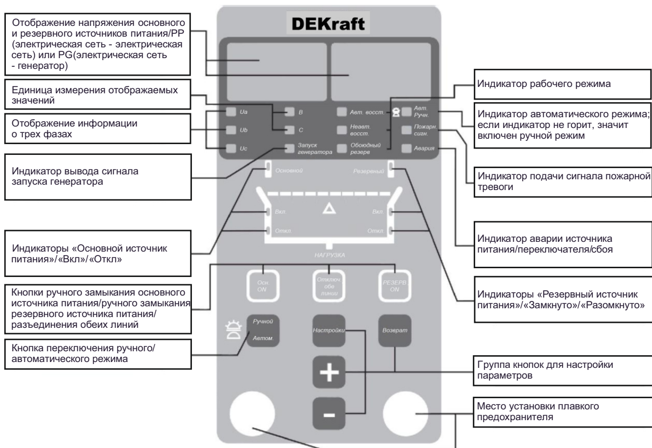
Рисунок 2. Лицевая панель контроллера блока.
