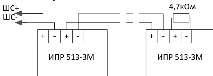
Рисунок 2.3. Схемы подключения извещателей в ШС прибора (продолжение)
