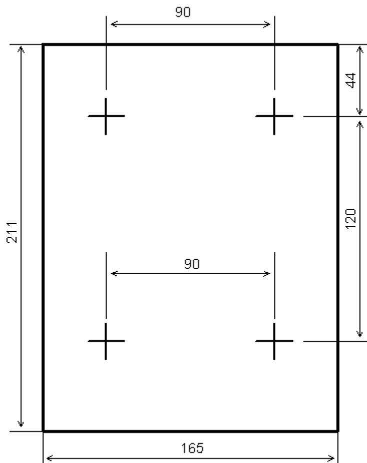
Рисунок 2.2.2.4-1 Габаритные и монтажные размеры
