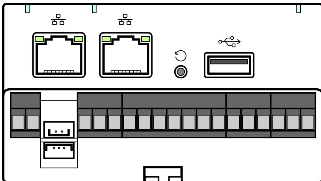
Схема расположения основных элементов на корпусе контроллера E2 Pro, вид сбоку.
