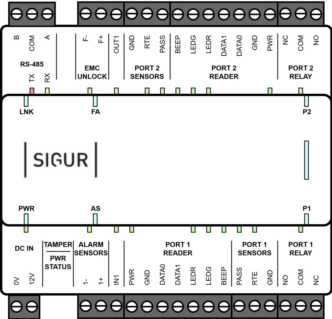
Схема расположения основных элементов на корпусе контроллера E2 Lite и E2 Pro, вид сверху.
