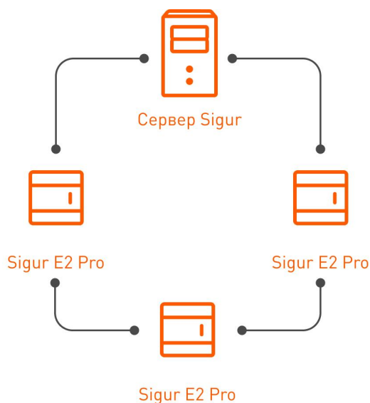
Пример подключения контроллеров E2 Pro по кольцевой топологии.
