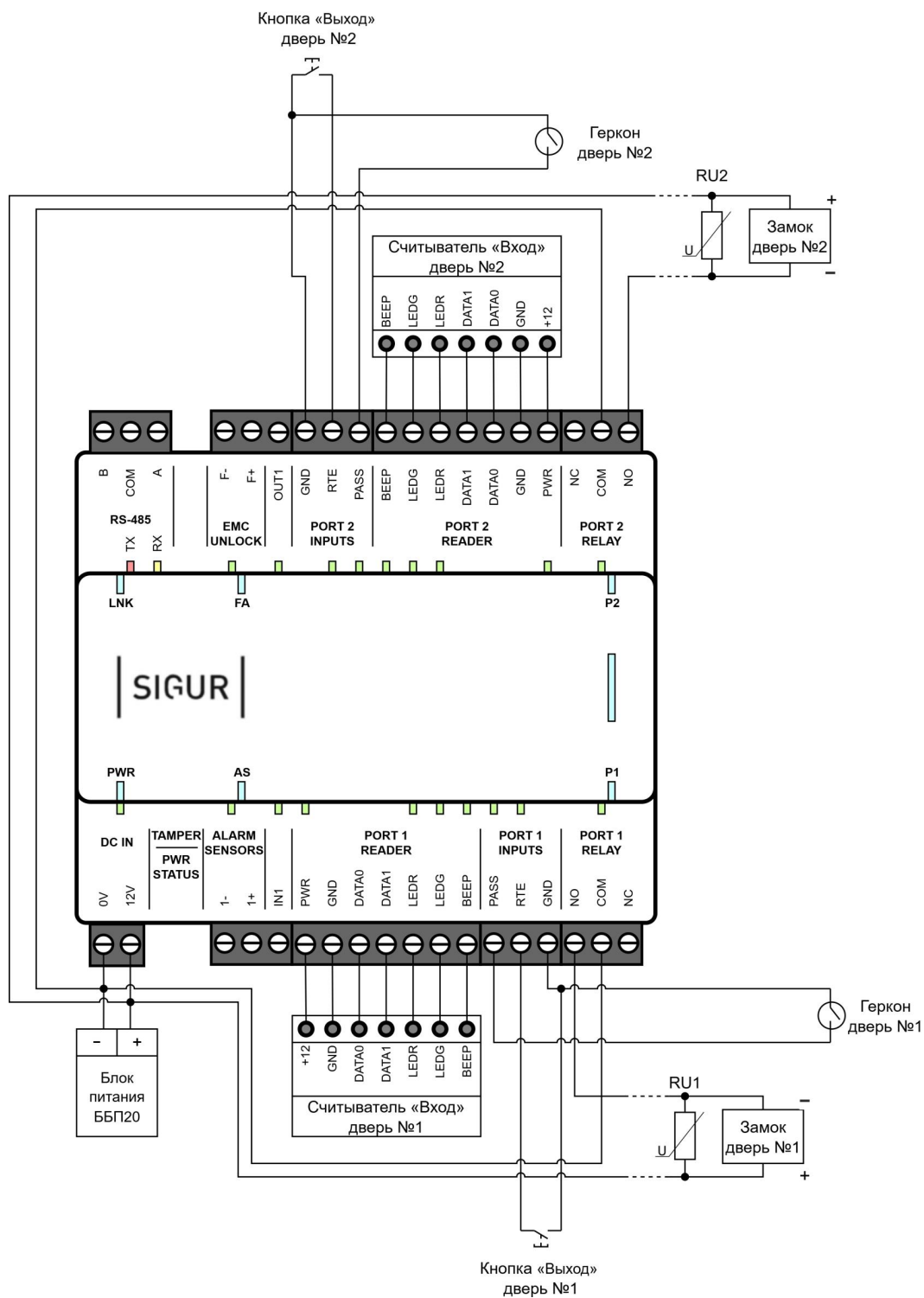
Пример подключения двух дверей.
