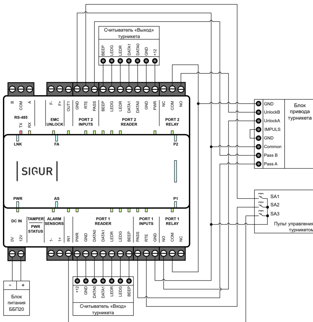
Пример подключения турникета.
