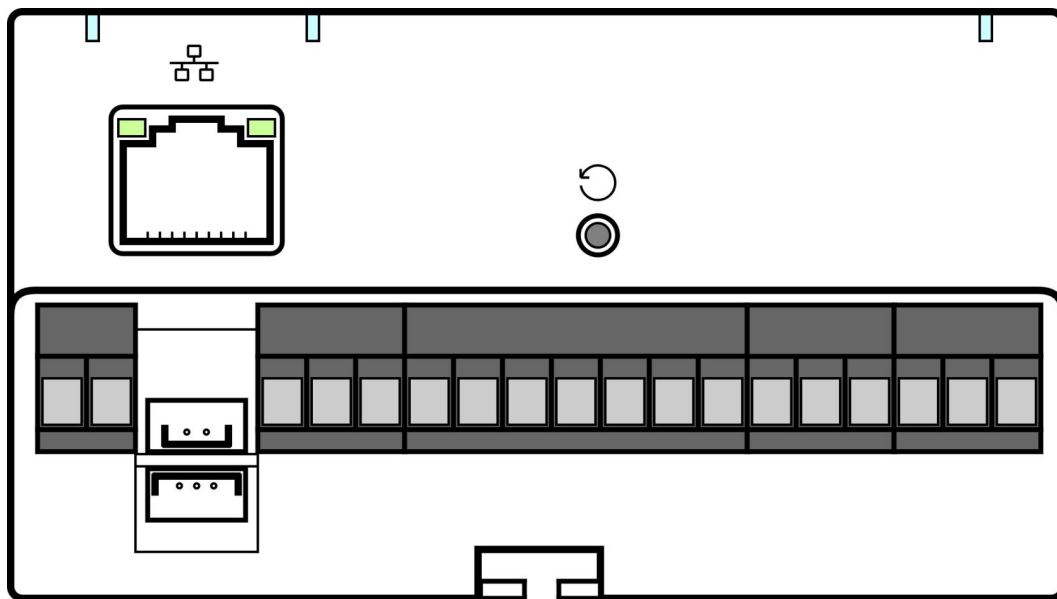
Схема расположения основных элементов на корпусе контроллера E2 Lite, вид сбоку.
