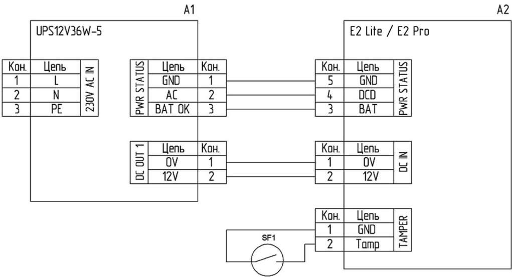
Схема электрическая принципиальная контроллера E2 Lite UPS и E2 Pro UPS.
