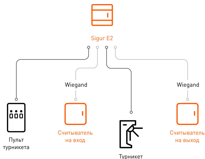
Вариант подключения в конфигурации «Турникет, потенциальное управление».
