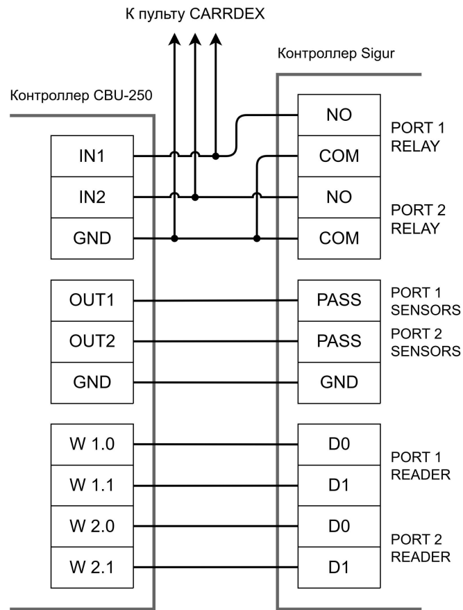
Электронные проходные CARDDEX, контроллер турникета CBU-250 (CBU-150/250).
