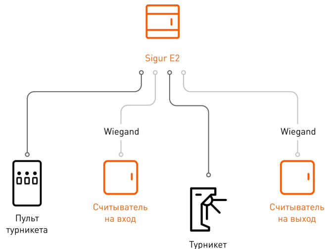
Вариант подключения в конфигурации «Турникет, потенциальное управление».
