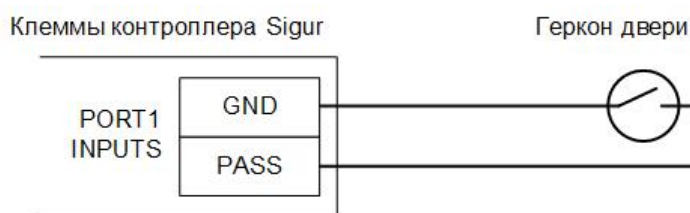
Подключение датчика открытия дверей.
