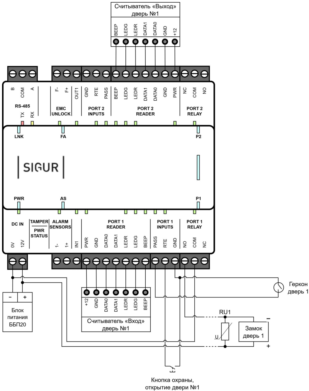
Пример подключения одной двери.
