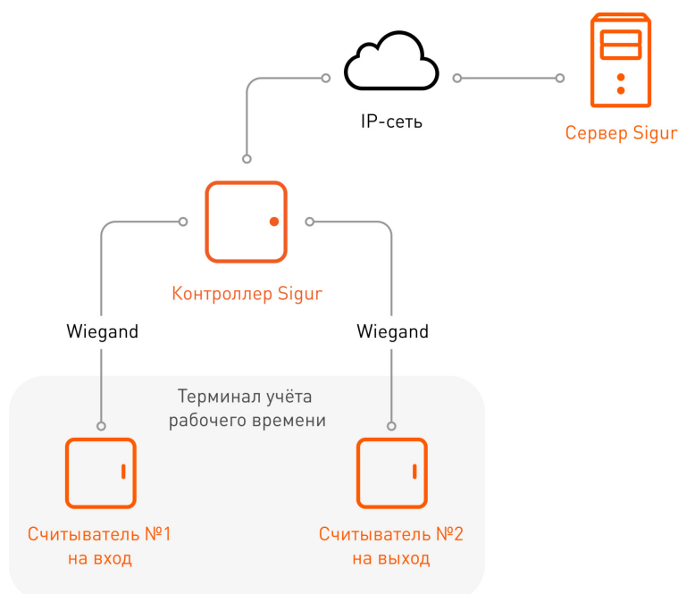
Вариант подключения в конфигурации «Терминал учёта рабочего времени».
