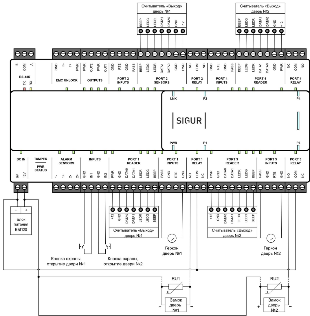
Пример подключения двух дверей.
