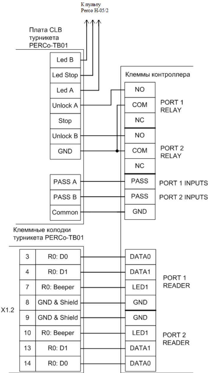
Подключение турникета PERCo TB-01.
