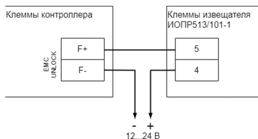
Подключение охранно-пожарного извещателя ИОПР513/101-1 к одному контроллеру.
