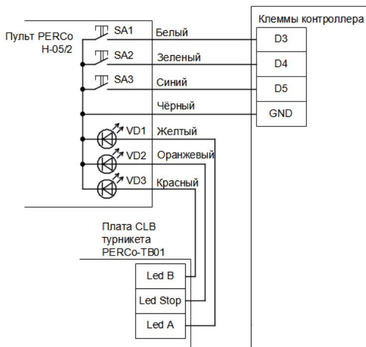
Подключение пульта PERCo H-05/2.
