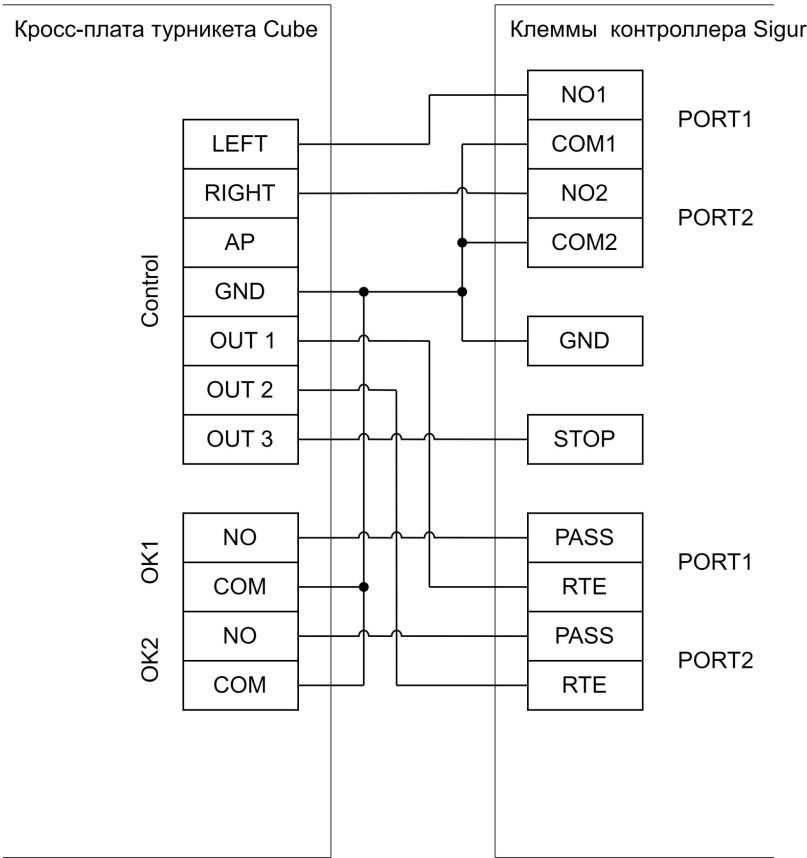
Подключение турникета Cube C-04.
