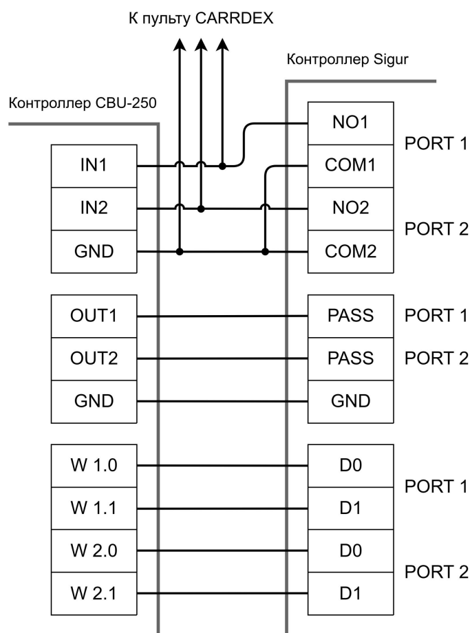
Электронные проходные CARDDEX, контроллер турникета CBU-250 (CBU-150/250).
