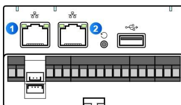
Нумерация Ethernet-портов на контроллере E2 Pro.
