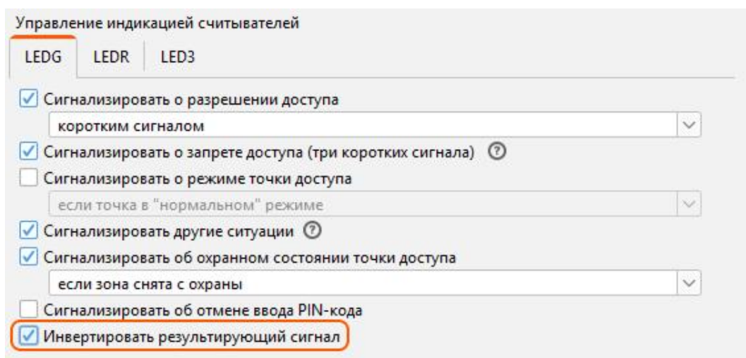
Пример настроек для выходов контроллера LEDG.
