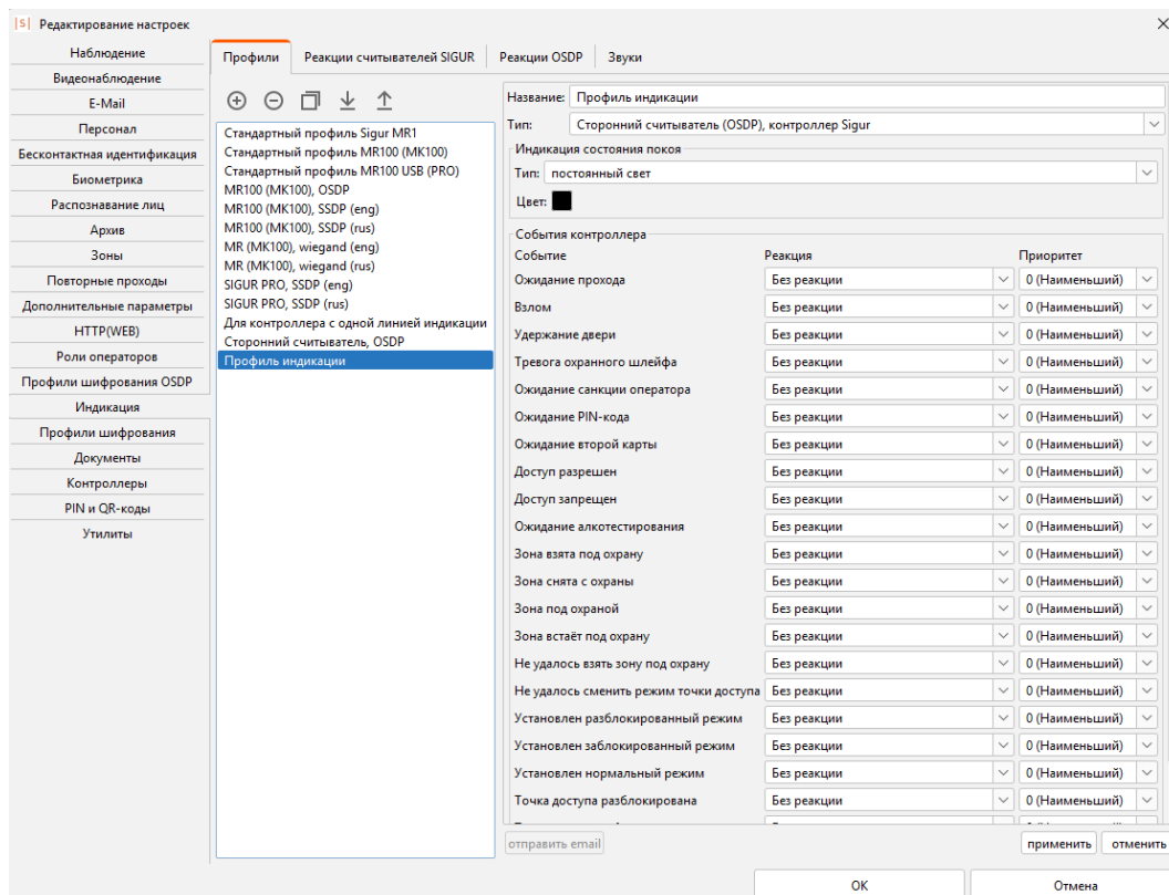
Создание нового профиля индикации для стороннего считывателя.
