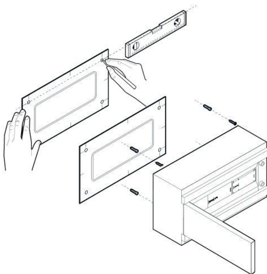
Монтаж контроллера.
