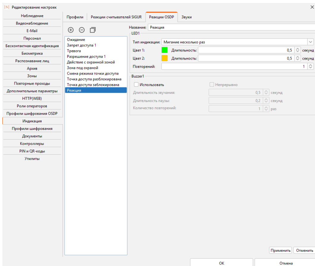
Создание реакции OSDP считывателя.
