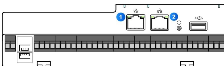
Нумерация Ethernet-портов на контроллере E4 Pro.
