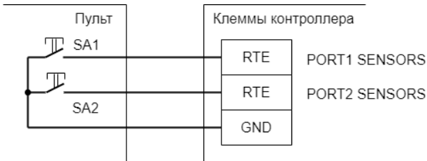
Пример подключения пульта ручного управления шлагбаумом/воротами к контроллеру, кнопка «Стоп» нормально разомкнута.
