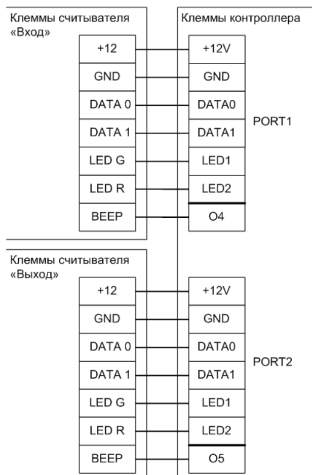
Пример подключения считывателей для PERCo-KT02 и KT05.3.
