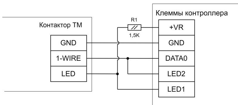
Пример подключения контактора Touch memory со встроенным светодиодом 1.
