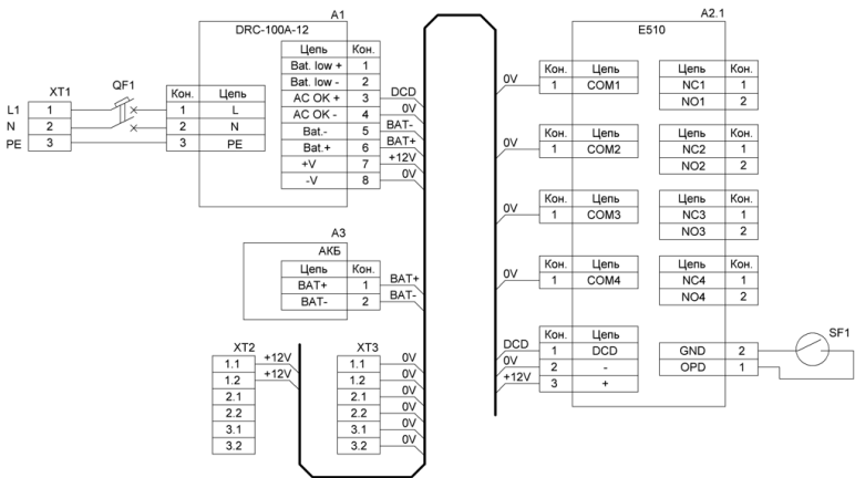
Схема электрическая принципиальная контроллера Sigur E510 UPS.
