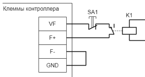
Подключение пожарной сигнализации и кнопки разблокировки к контроллеру.
